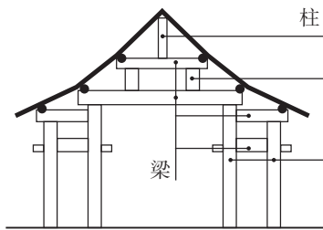
中国古建筑大木构架剖面示意图
